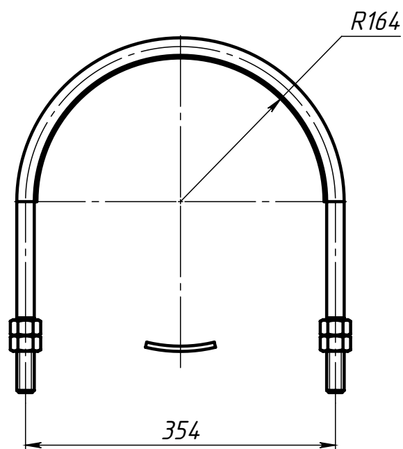
Поз.1 (Хомут)
