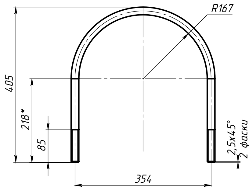
Поз.1 (Хомут)
